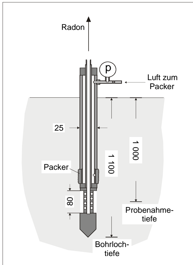
Abb. A1.3 Skizze einer Bodenluftsonde (nicht maßstabsgerecht, Bemaßung in Millimeter)
