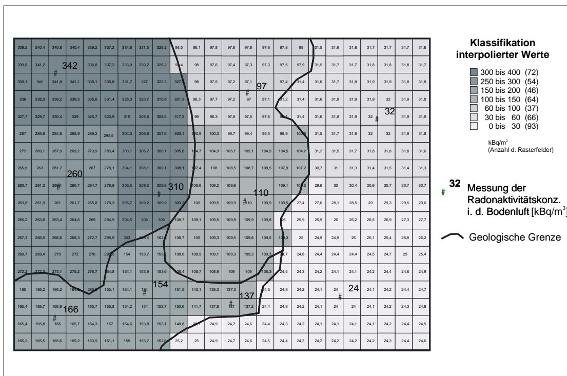
Abb. A1.5 Abstandsgewichtete Interpolation der Radonaktivitätskonzentration in der Bodenluft unter Berücksichtigung geologischer Grenzen
